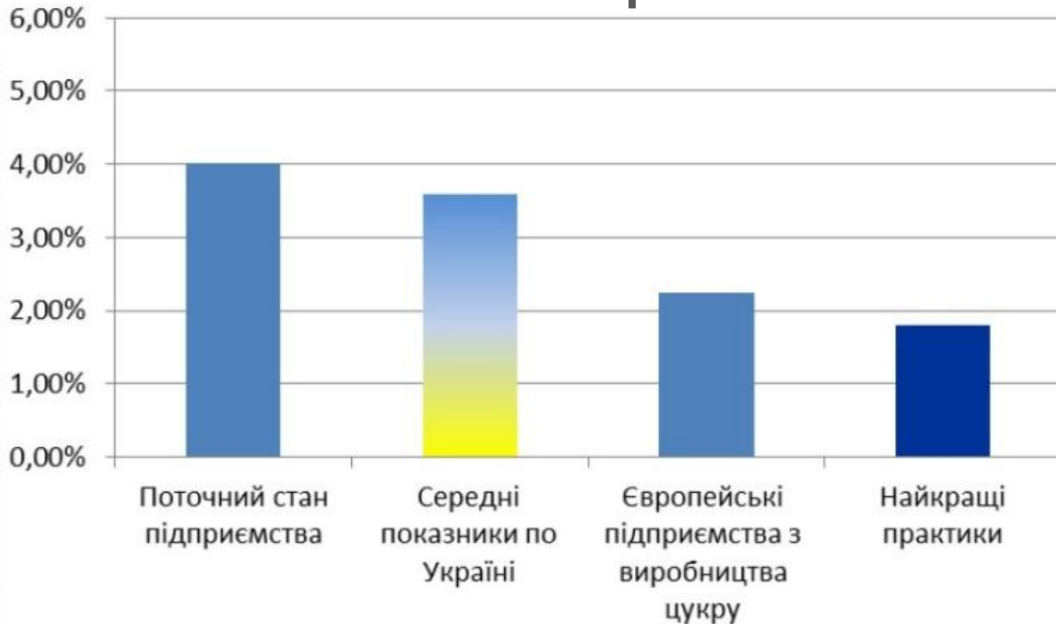
Рис.1. Питомі показники споживання енергоресурсів на 1 т переробленого буряку (без витрат на газову піч)
