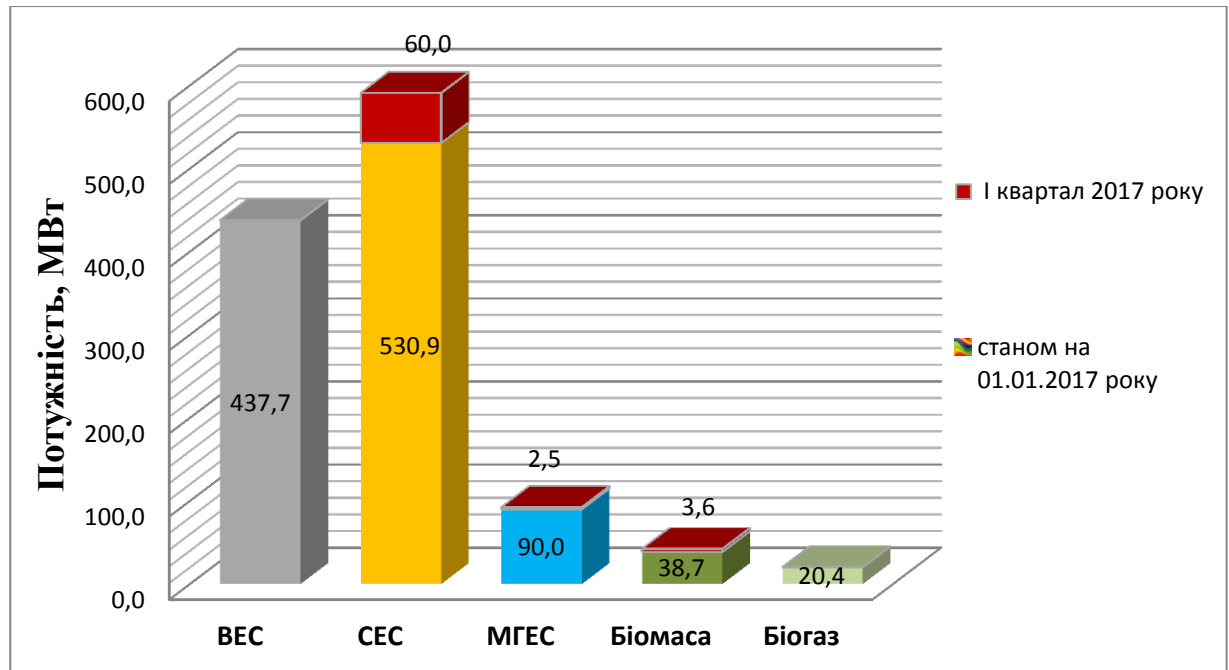
Потужність об'єктів відновлюваної електроенергетики, яким видано «зелений» тариф
